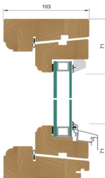
Snittritning
