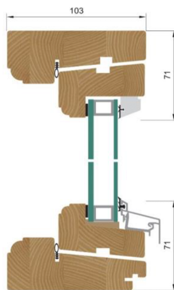
Snittritning
