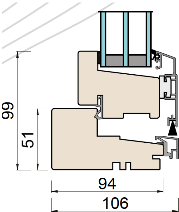
Snittritning
