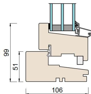
Snittritning
