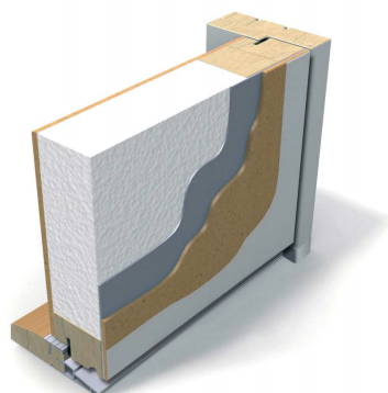
Genomskärning
